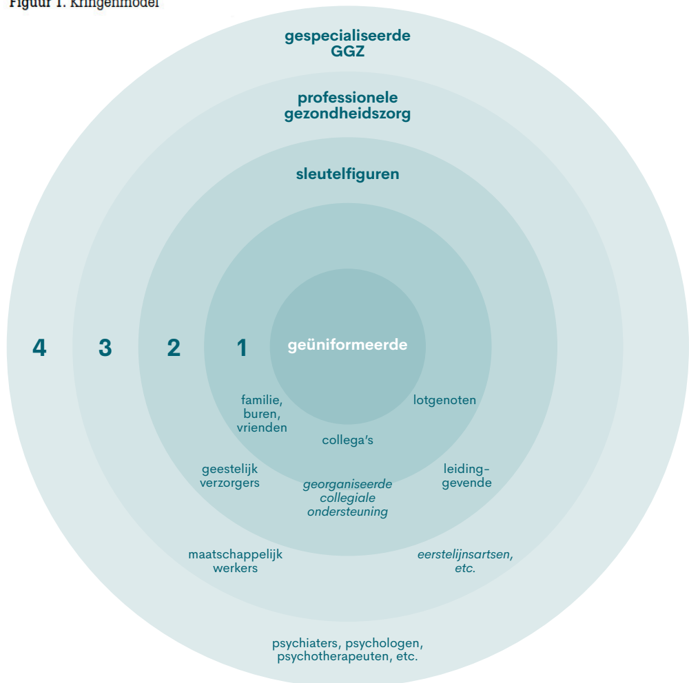
Figuur 1. Kringenmodel
